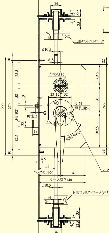
ロッドガイド正面図
